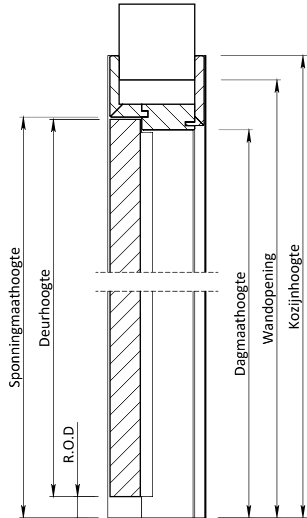
DOORSNEDE B-B
