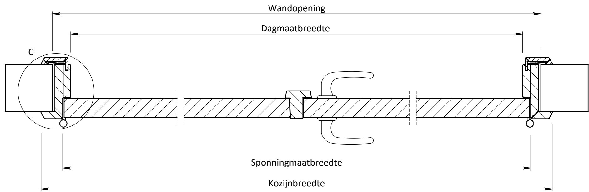
DOORSNEDE A-A
