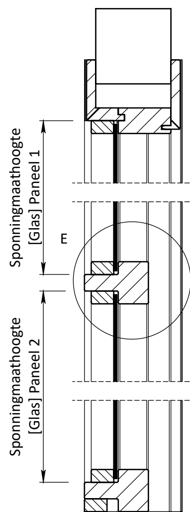
DOORSNEDE C-C
