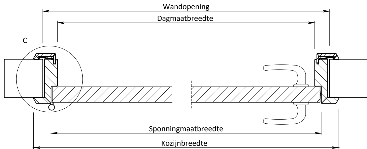
DOORSNEDE A-A
