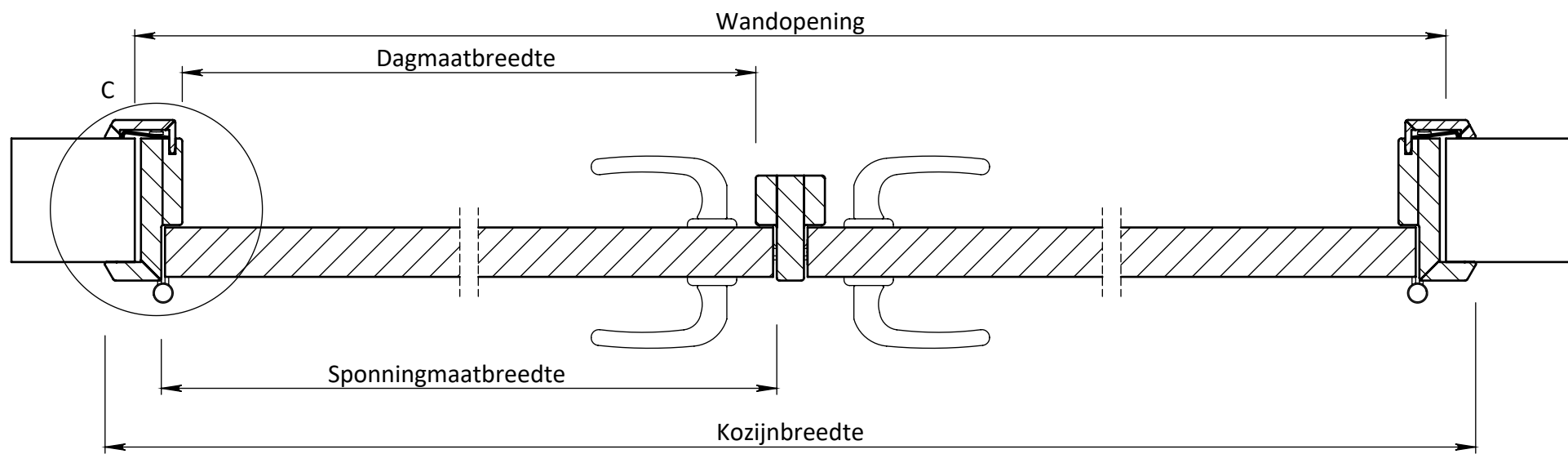
DOORSNEDE A-A
