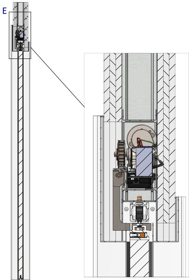
SECTION D-D
