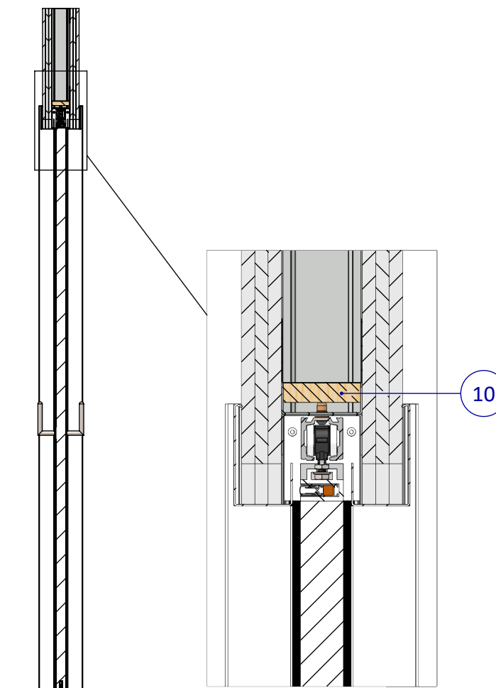
SECTION D-D
