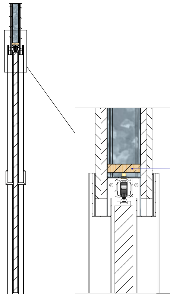
SECTION D-D
