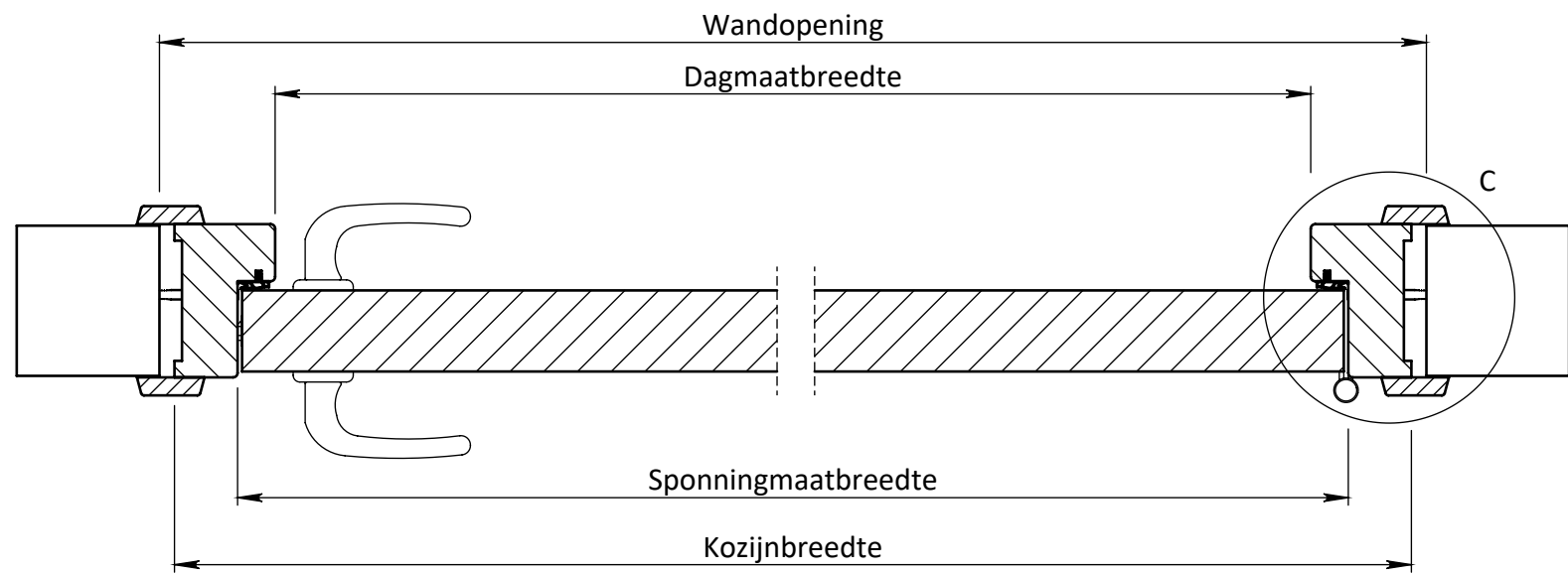
DOORSNEDE A-A
