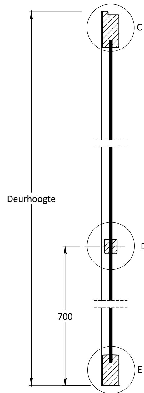
DOORSNEDE B-B
