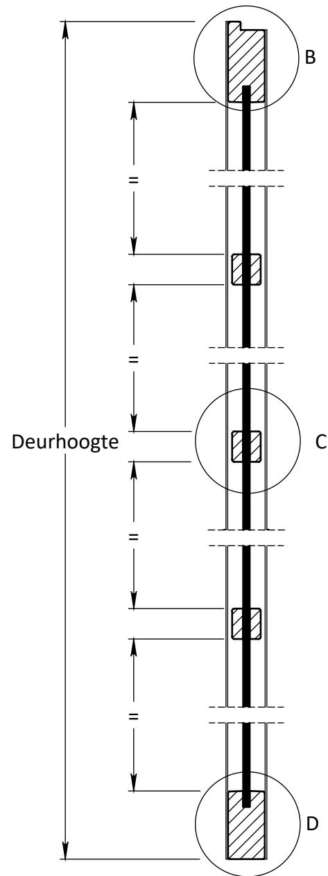
DOORSNEDE B-B
