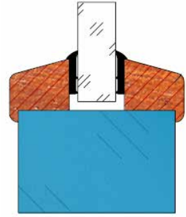
Doorsnede Slim Frame
