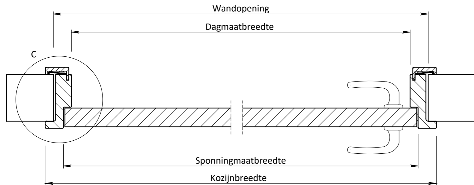
DOORSNEDE A-A
