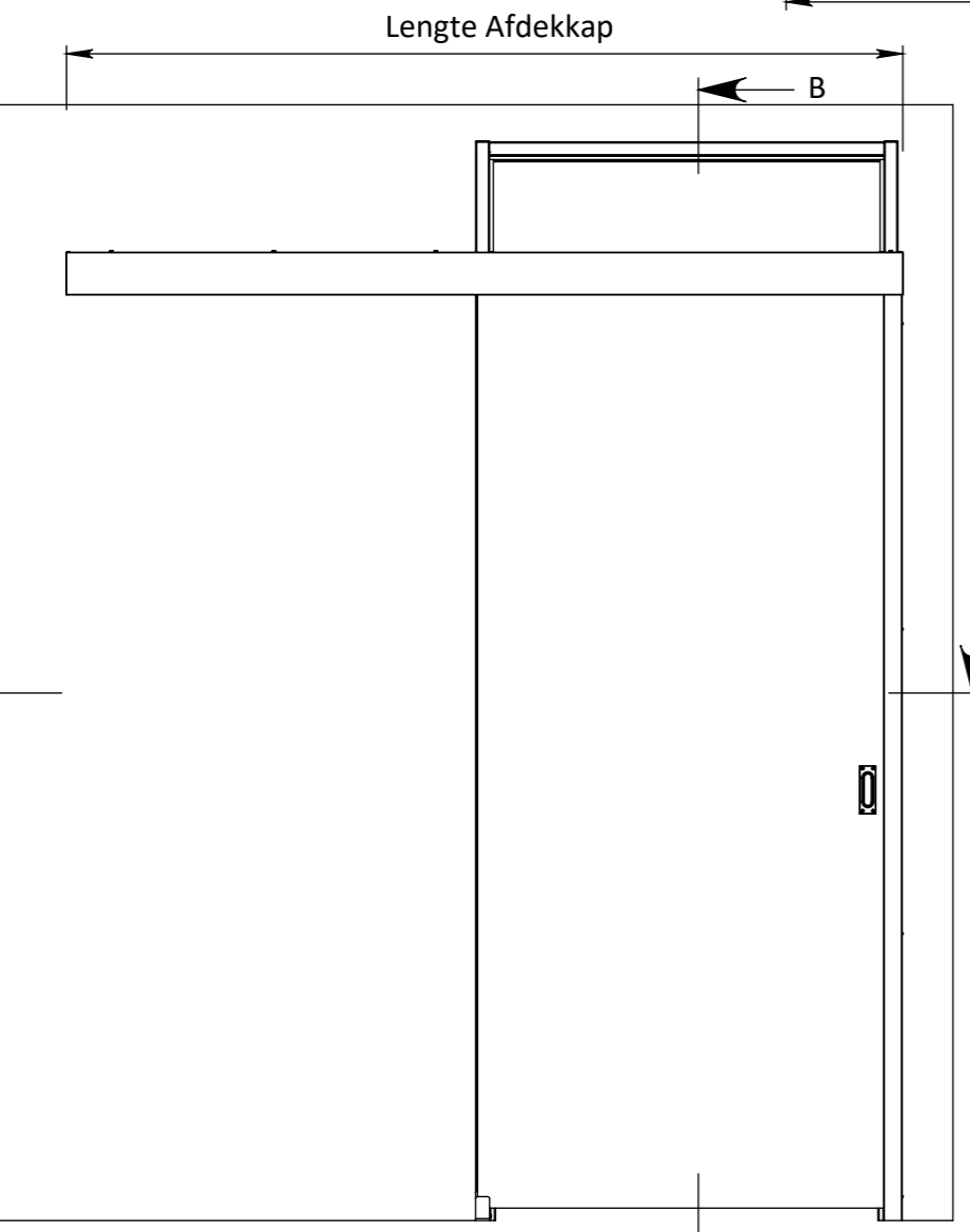
VOORAANZICHT
