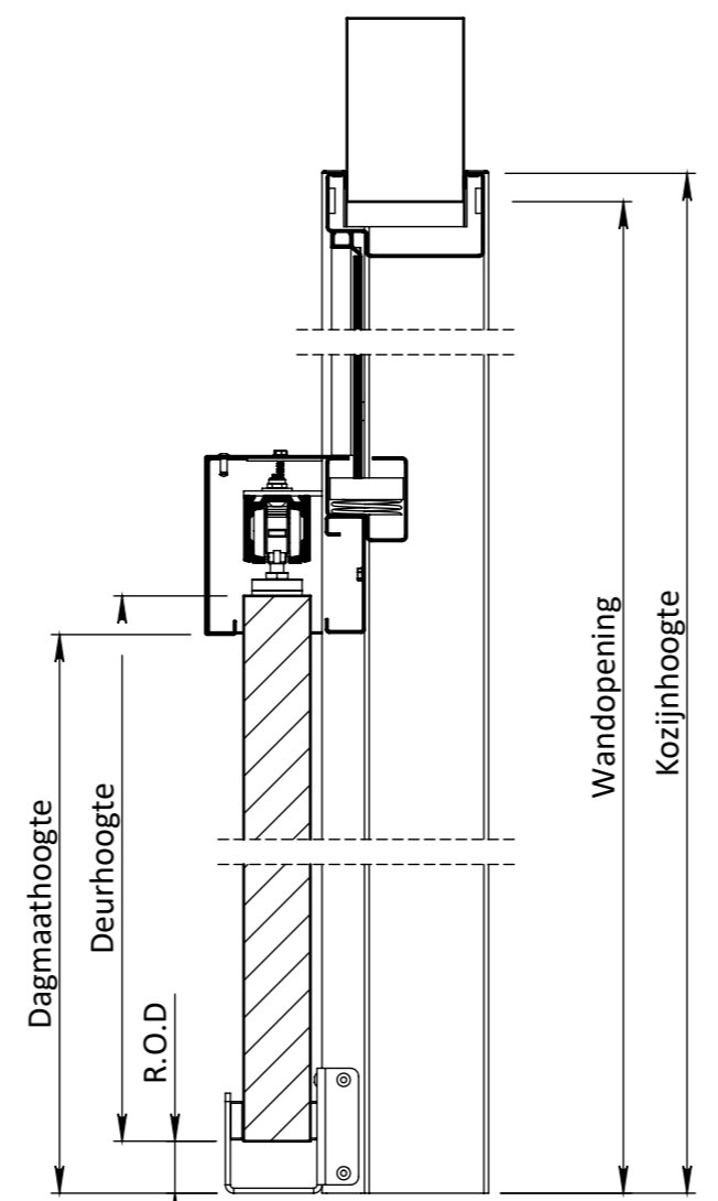
DOORSNEDE B-B
