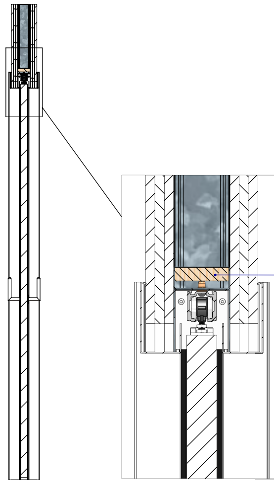
SECTION D-D
