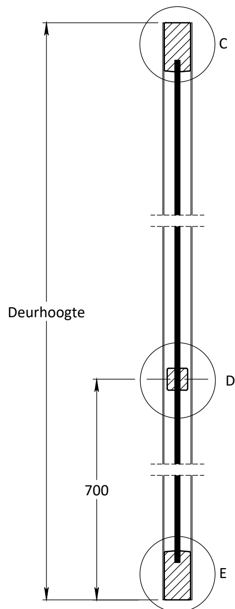
DOORSNEDE B-B
