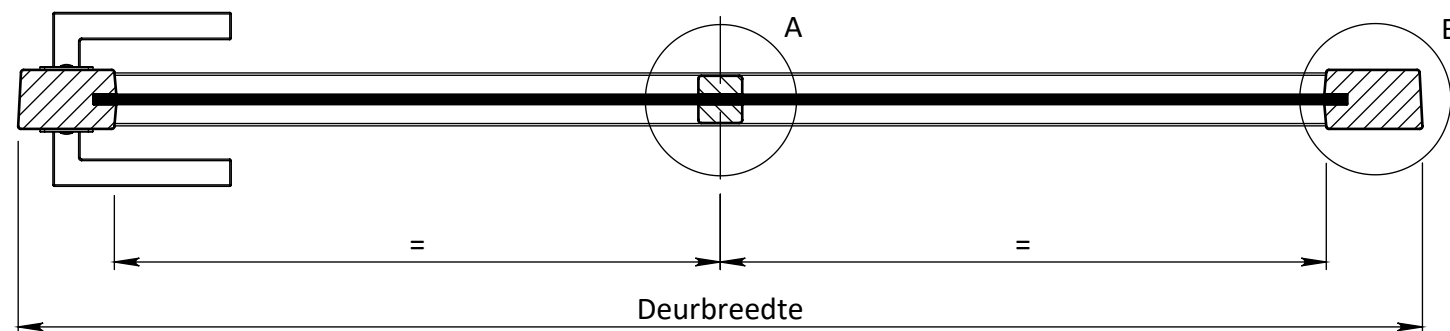
DOORSNEDE A-A
