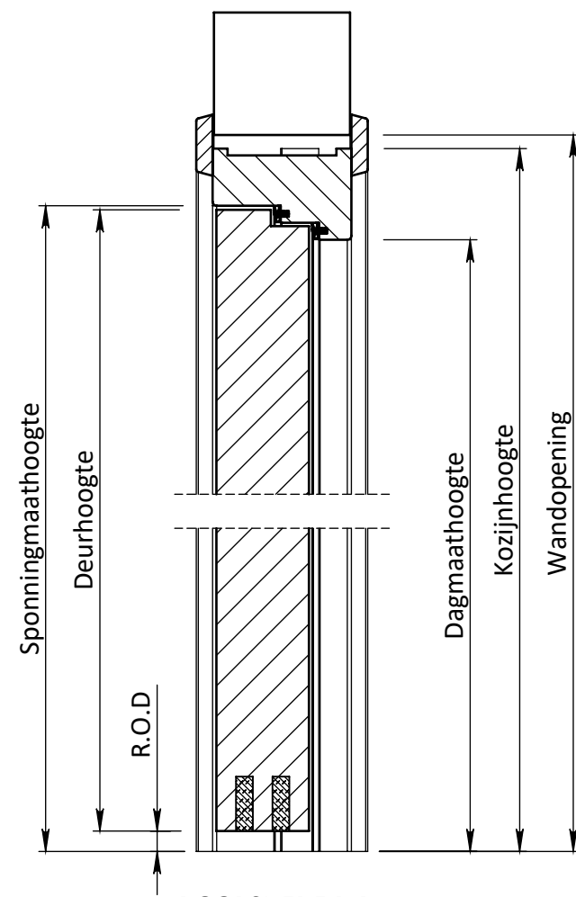
DOORSNEDE B-B
