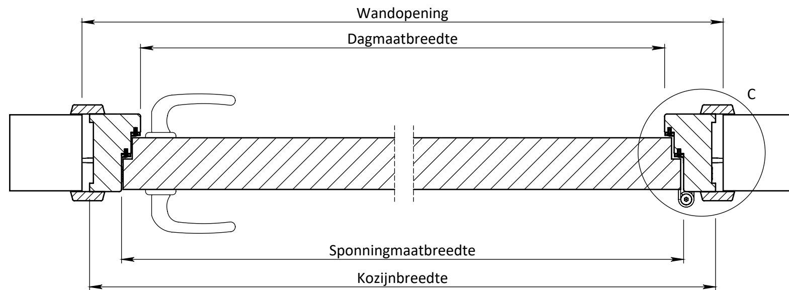
DOORSNEDE A-A
