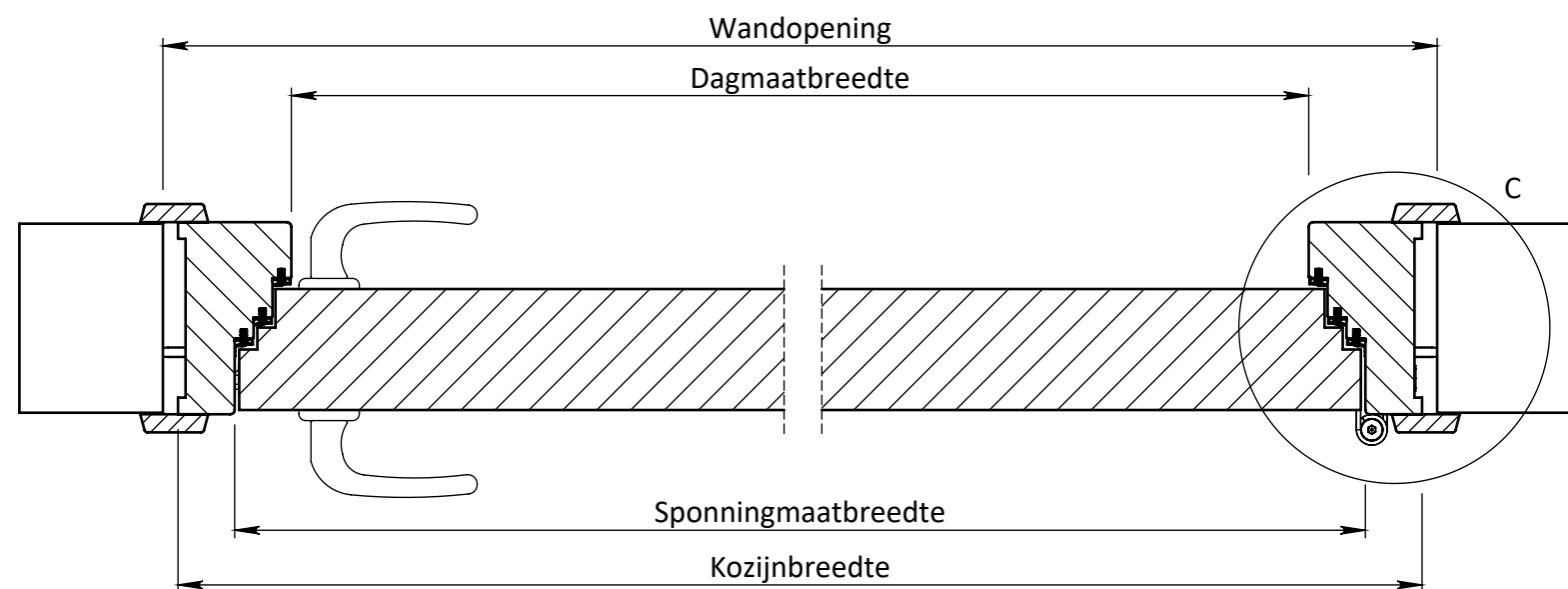
DOORSNEDE A-A
