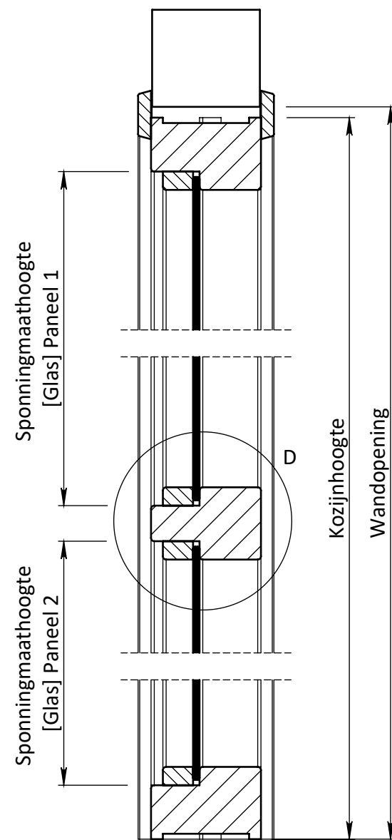
DOORSNEDE B-B
