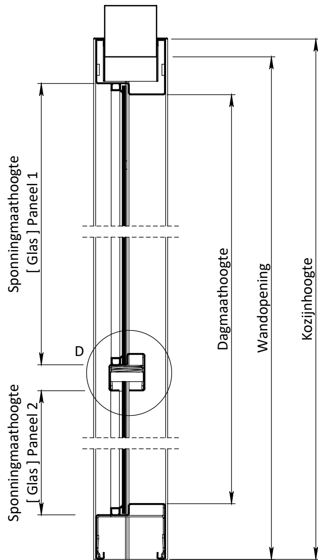
DOORSNEDE B-B
