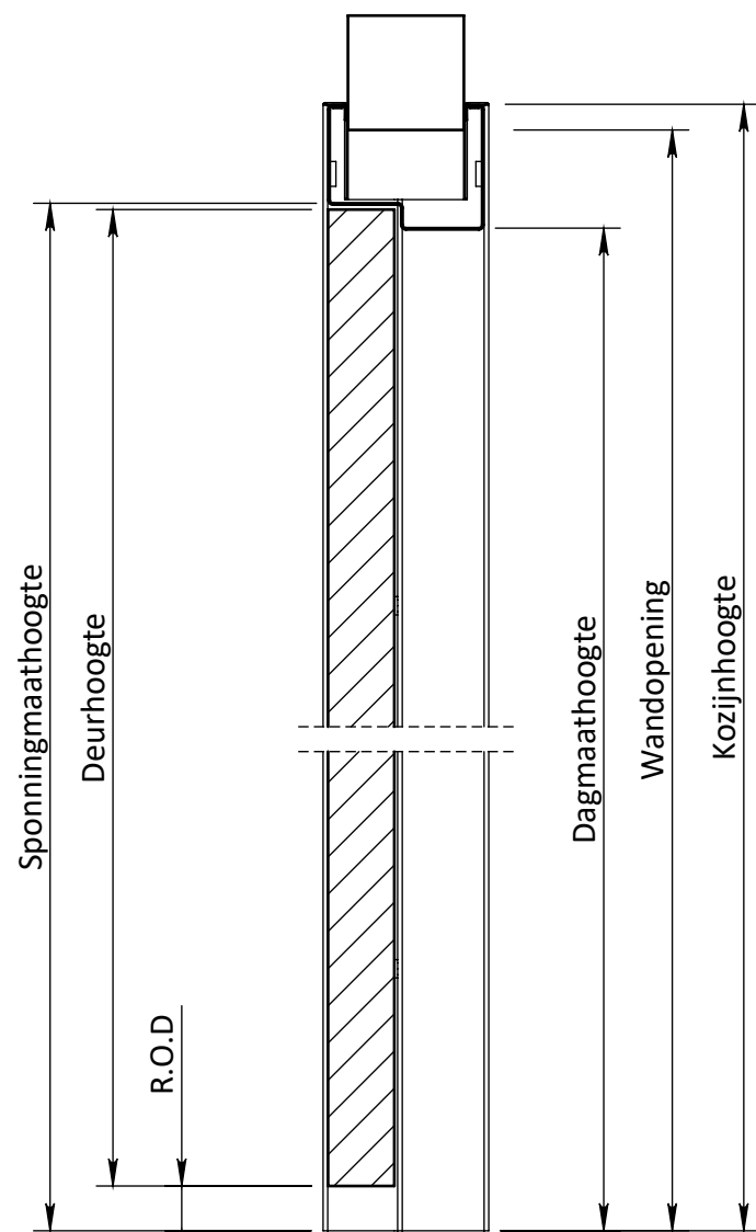
DOORSNEDE B-B
