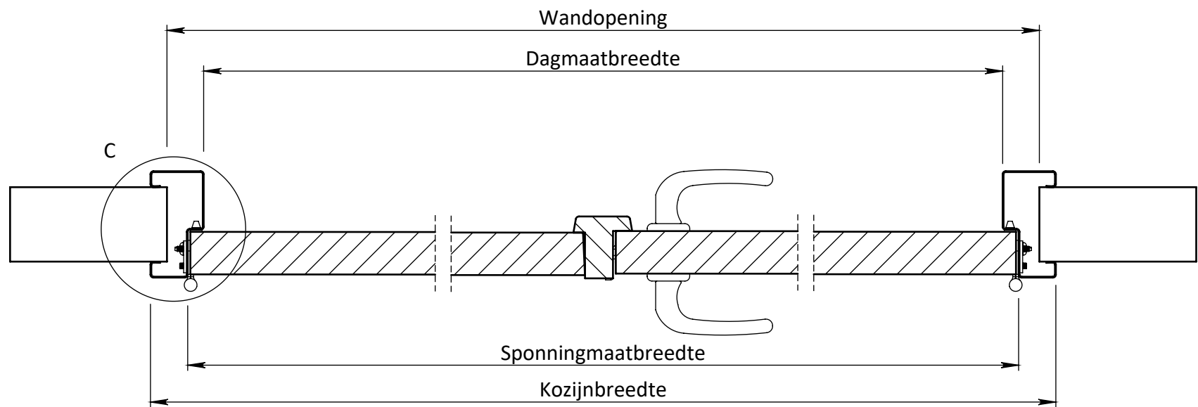
DOORSNEDE A-A
