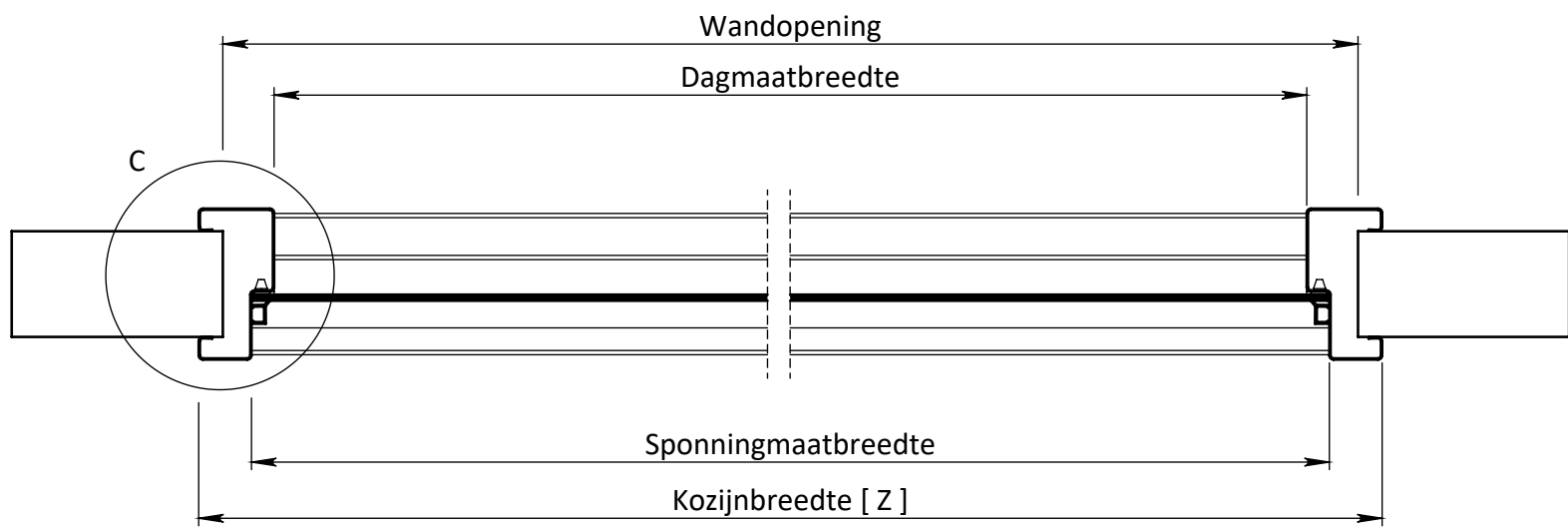
DOORSNEDE A-A
