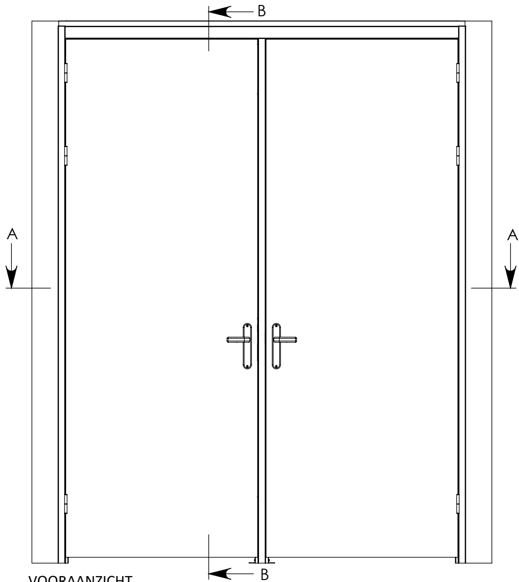
VOORAANZICHT
