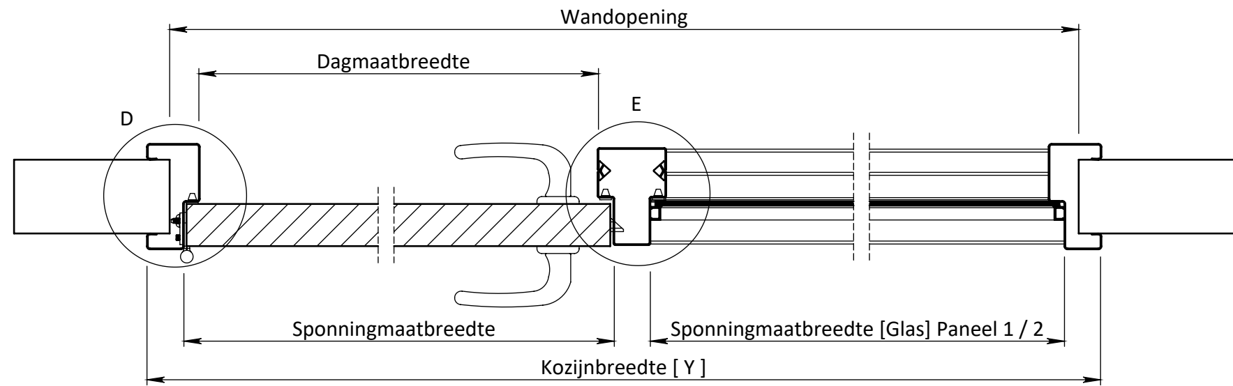
DOORSNEDE A-A
