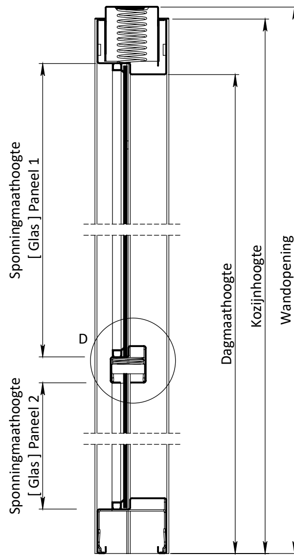
DOORSNEDE B-B
