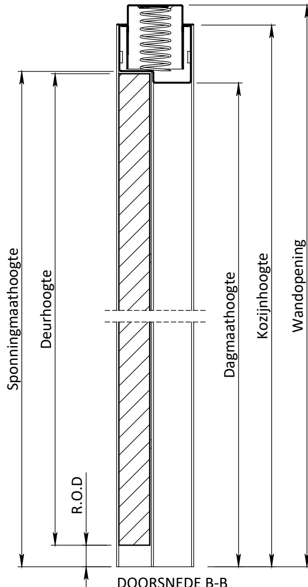
DOORSNEDE B-B
