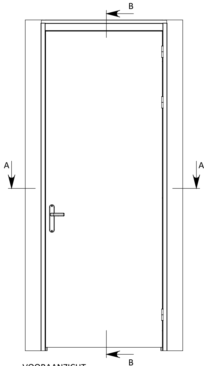
VOORAANZICHT
