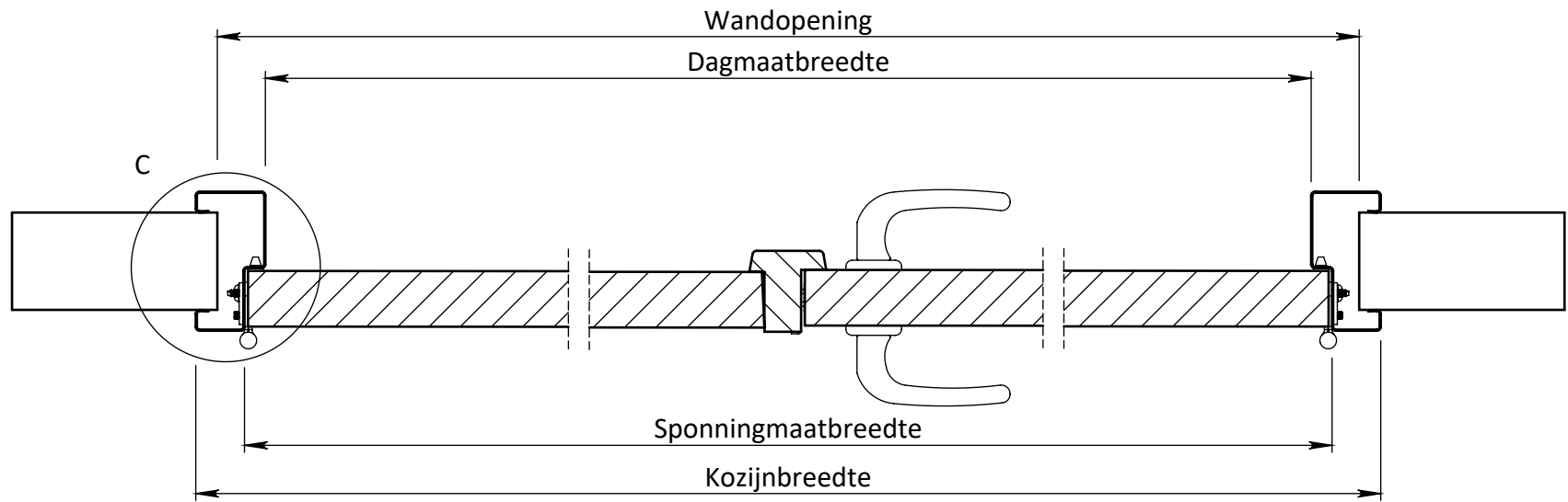
DOORSNEDE A-A
