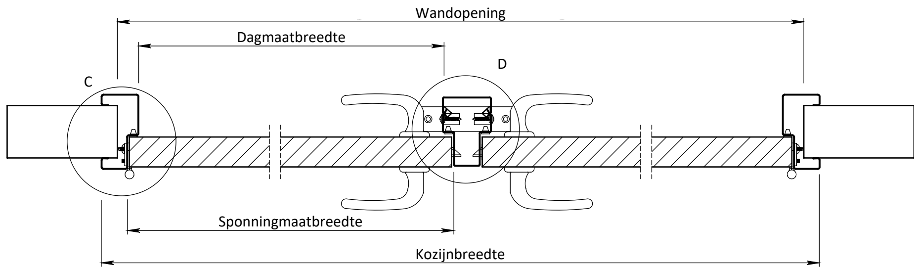
DOORSNEDE A-A
