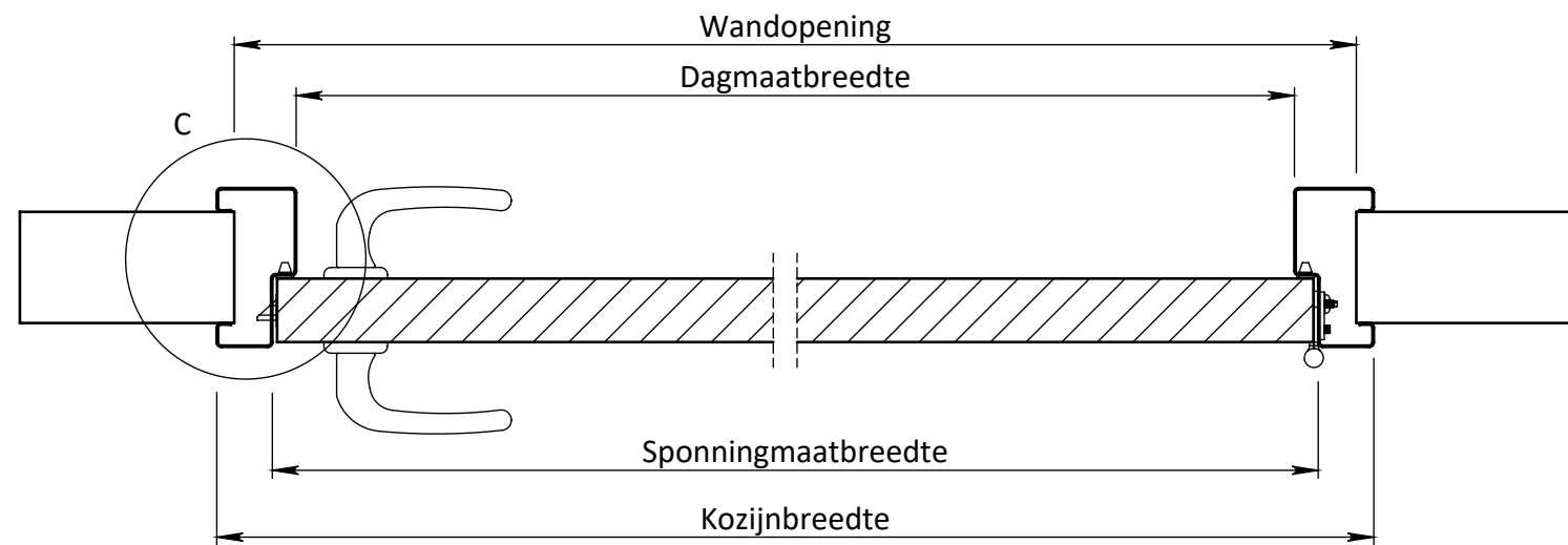
DOORSNEDE A-A
