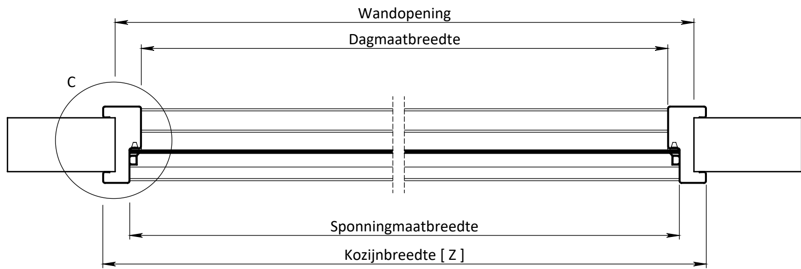
DOORSNEDE A-A
