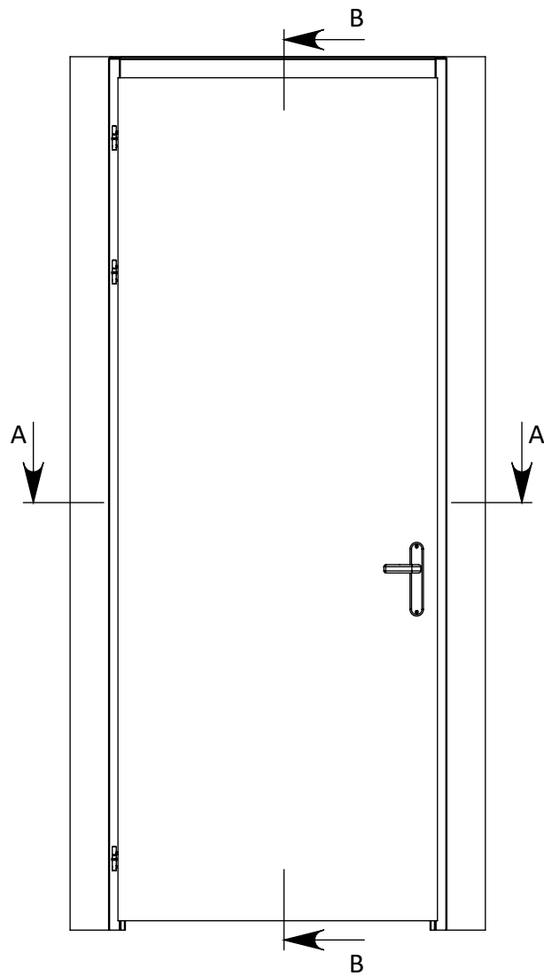
VOORAANZICHT
