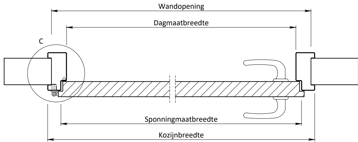
DOORSNEDE A-A
