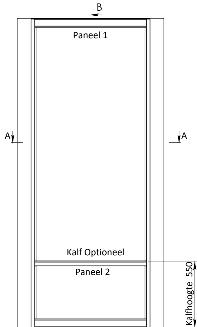
VOORAANZICHT
