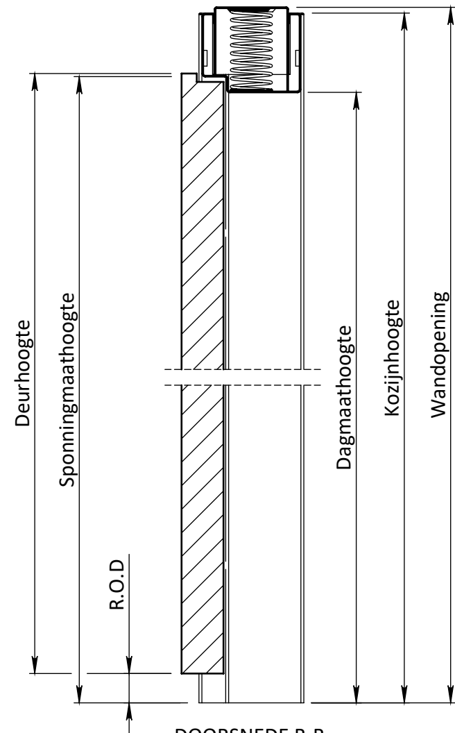
DOORSNEDE B-B
