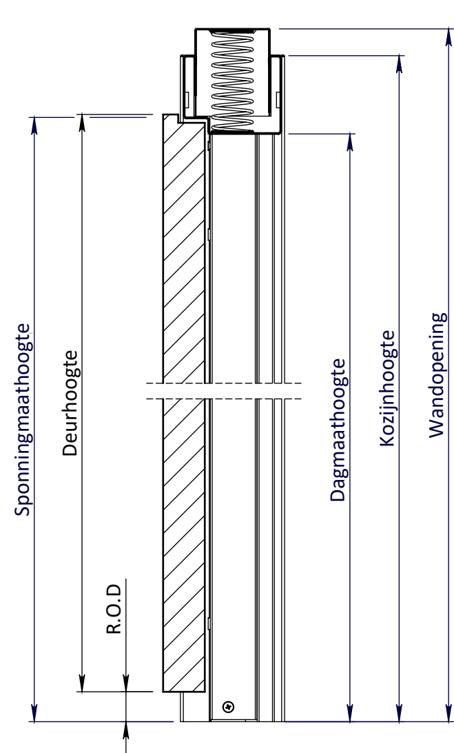
DOORSNEDE B-B
