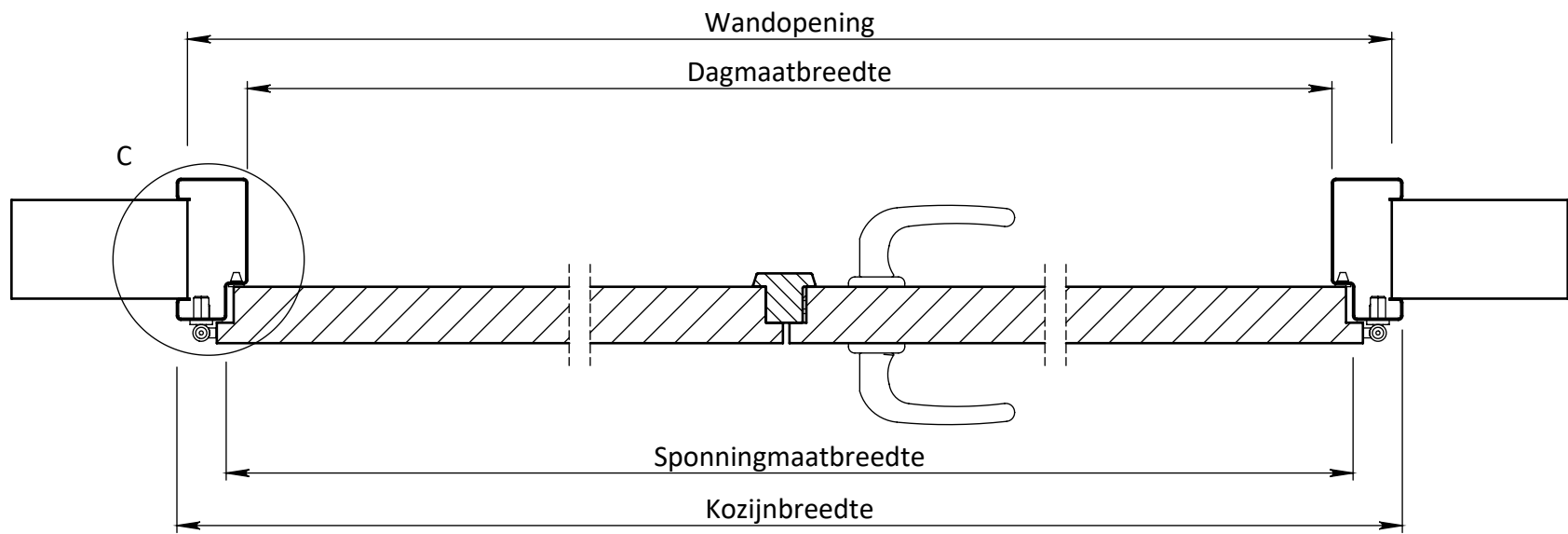
DOORSNEDE A-A
