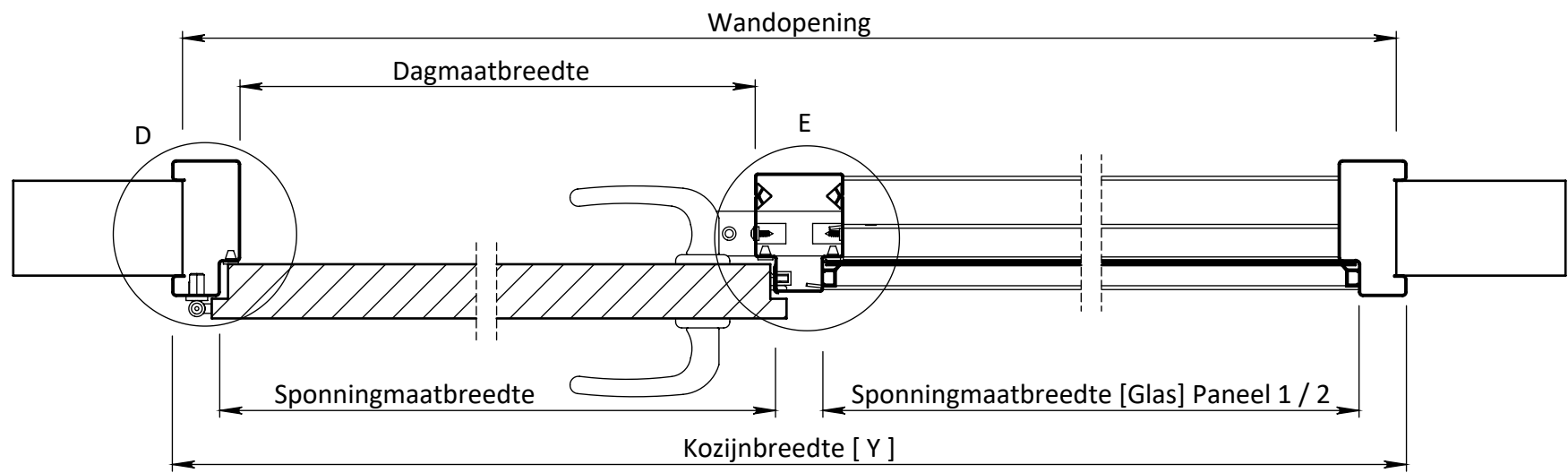
DOORSNEDE A-A
