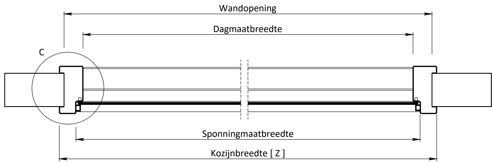
DOORSNEDE A-A
