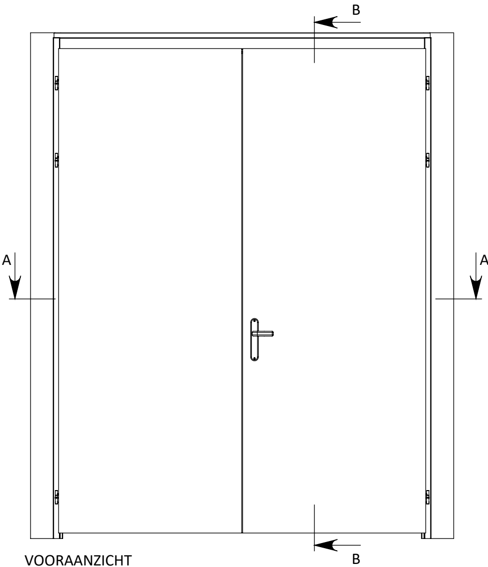
VOORAANZICHT
