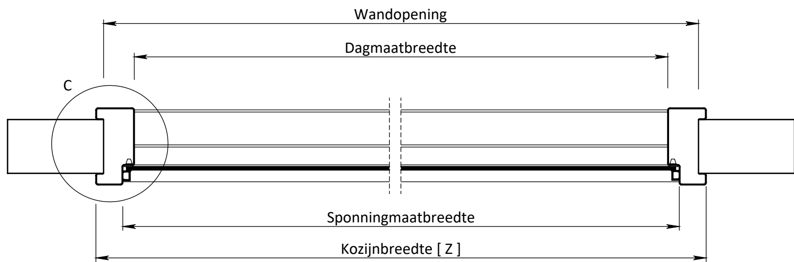
DOORSNEDE A-A
