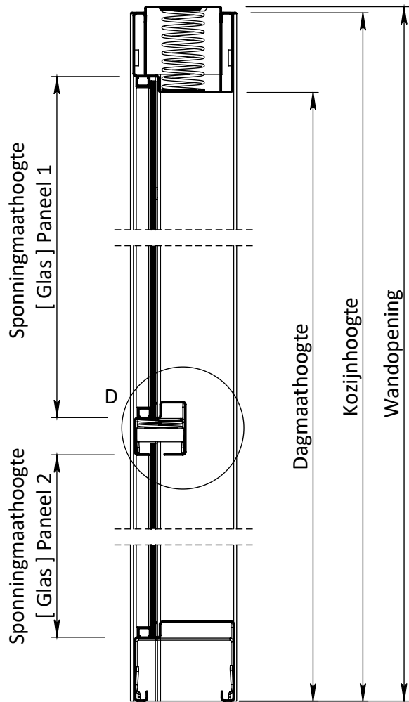
DOORSNEDE B-B
