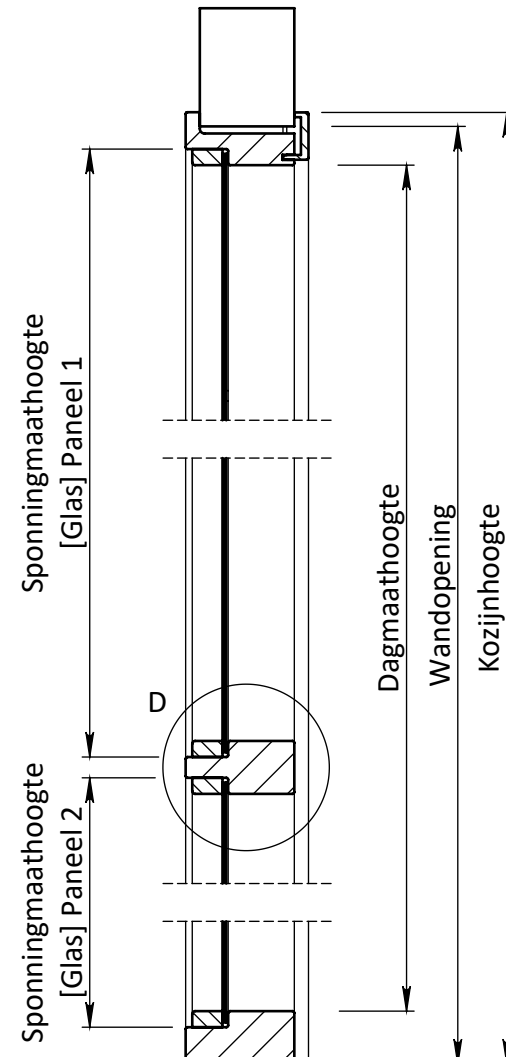
DOORSNEDE B-B
