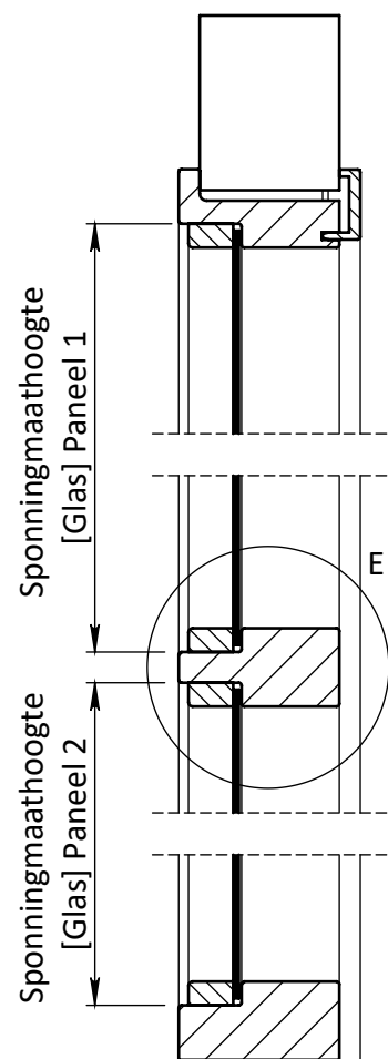
DOORSNEDE B-B
