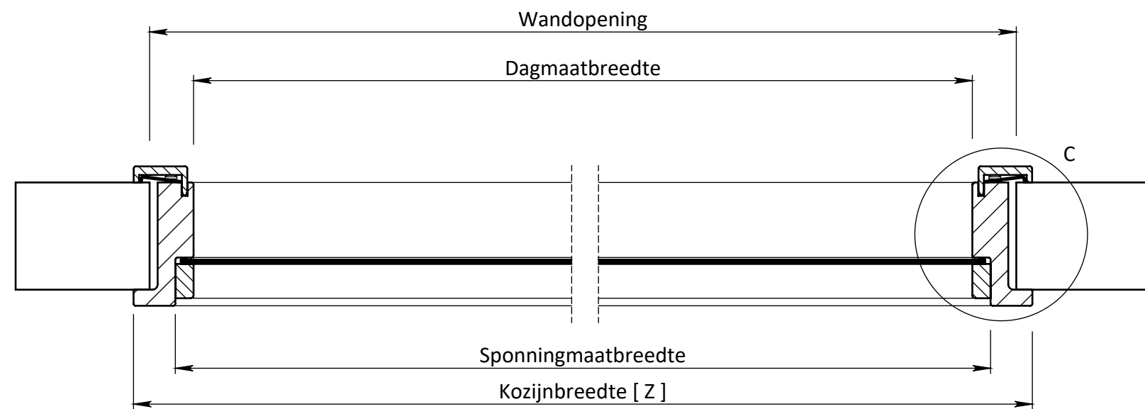
DOORSNEDE A-A
