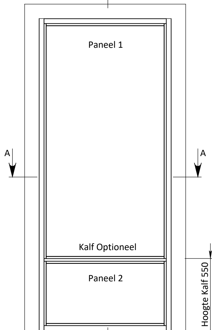
VOORAANZICHT
