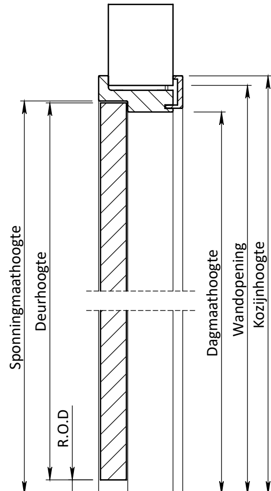
DOORSNEDE C-C
