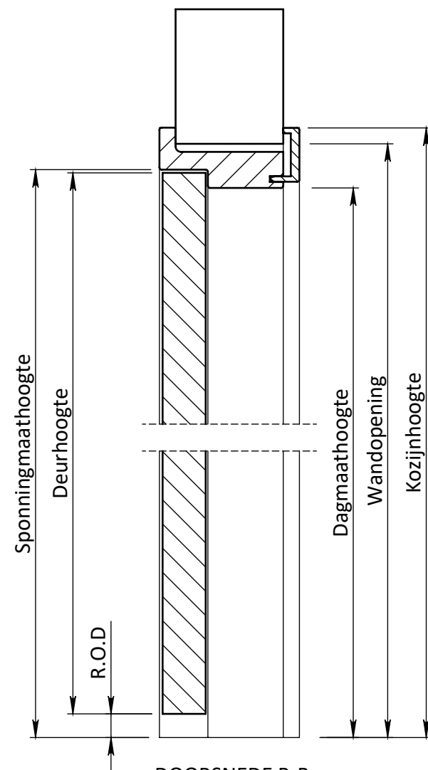
DOORSNEDE B-B
