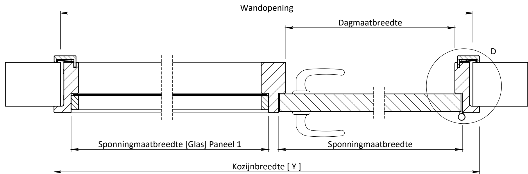
DOORSNEDE A-A
