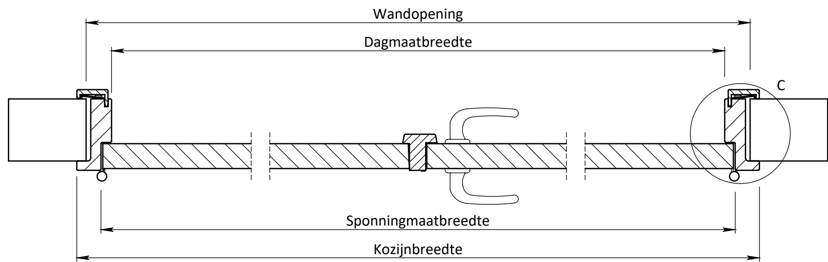
DOORSNEDE A-A
