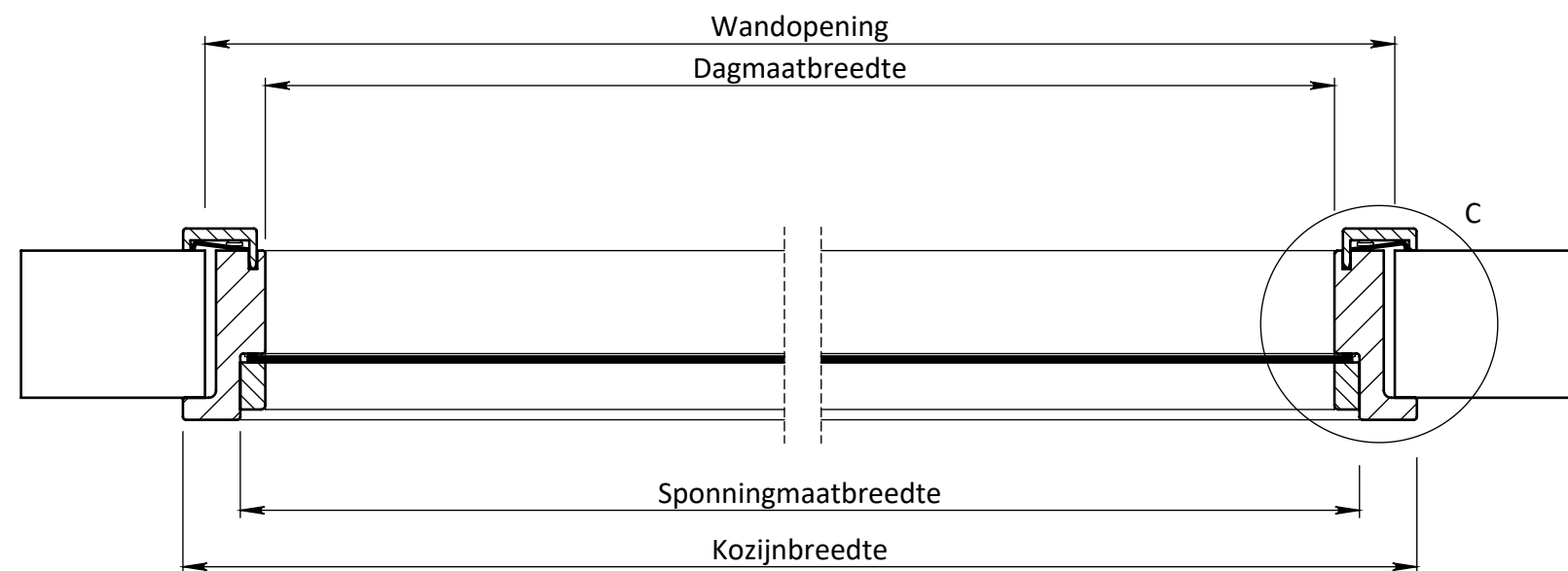
DOORSNEDE A-A
