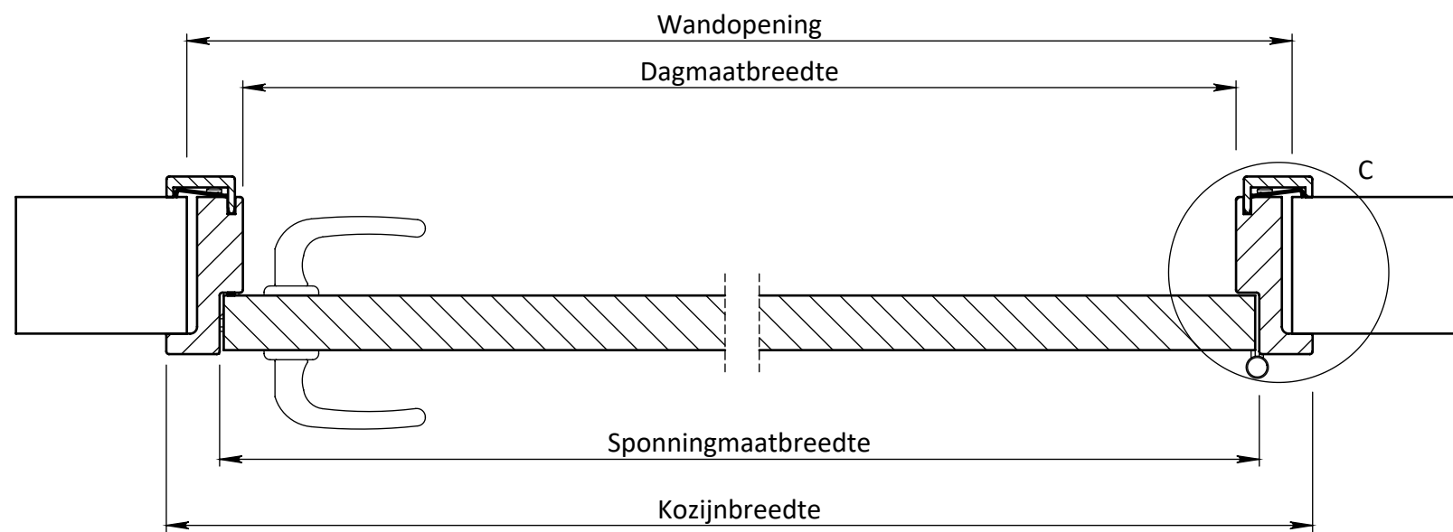
DOORSNEDE A-A
