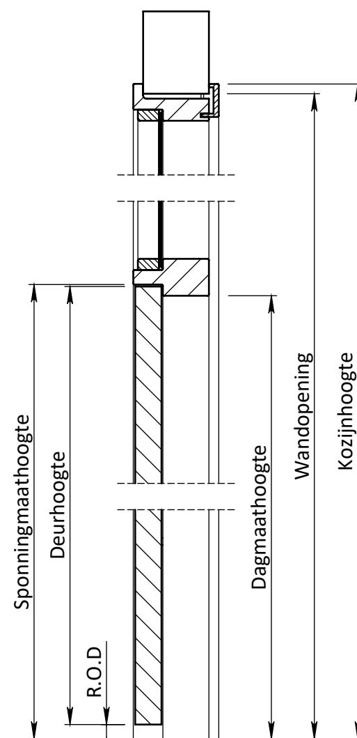
DOORSNEDE C-C
