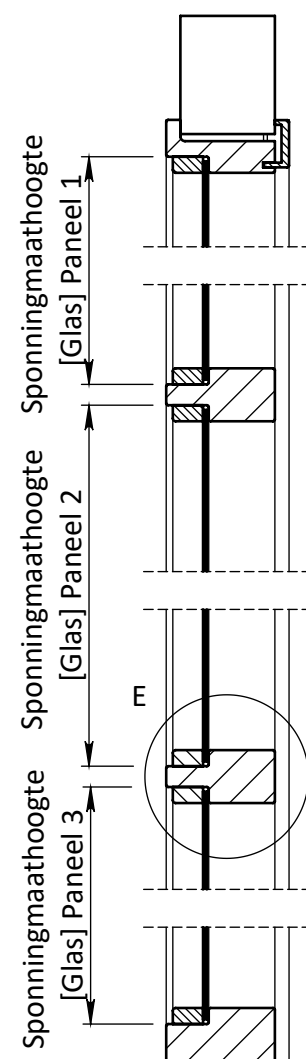
DOORSNEDE B-B
