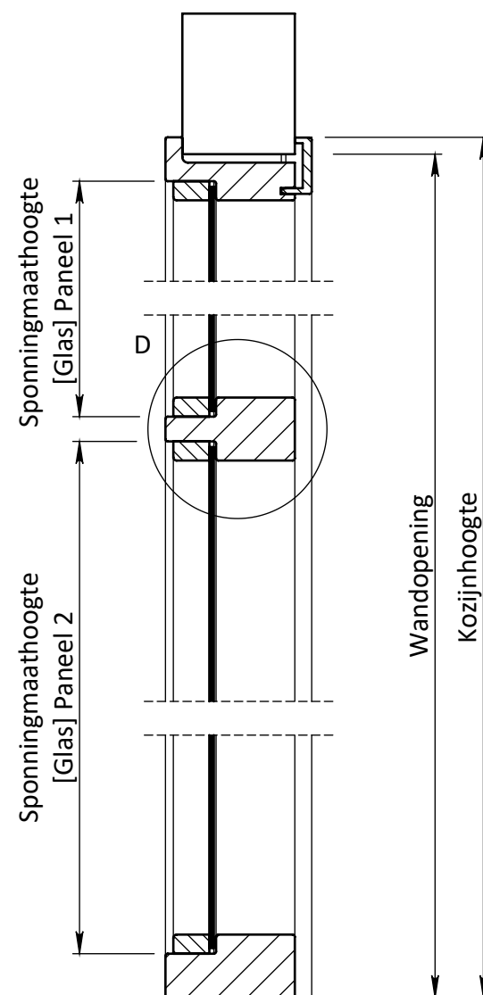
DOORSNEDE B-B
