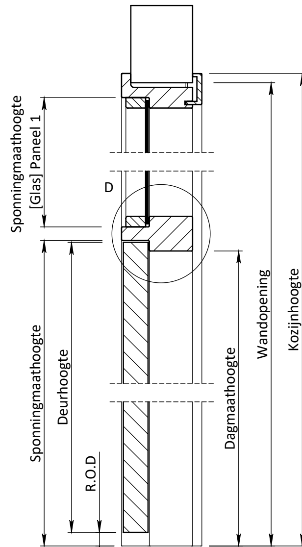
DOORSNEDE B-B
