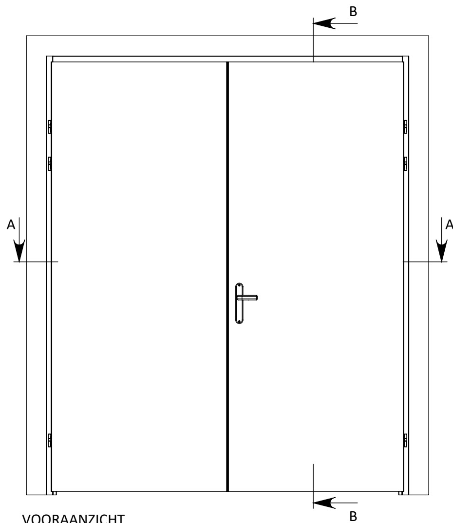
VOORAANZICHT
