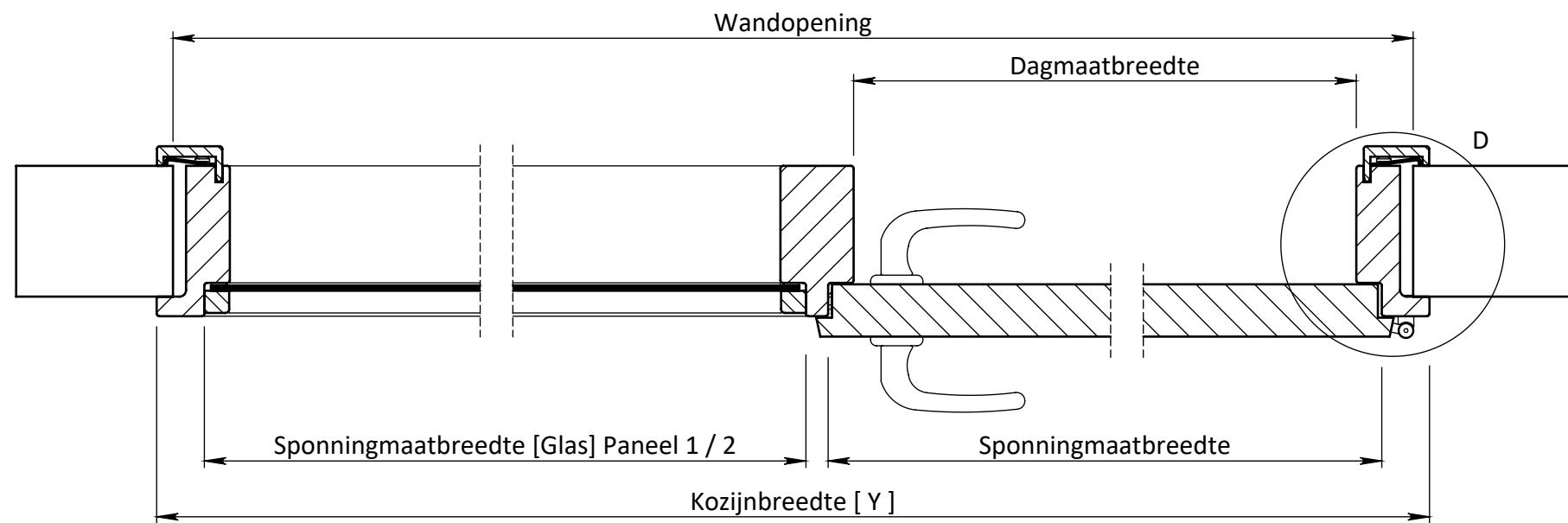
DOORSNEDE A-A
