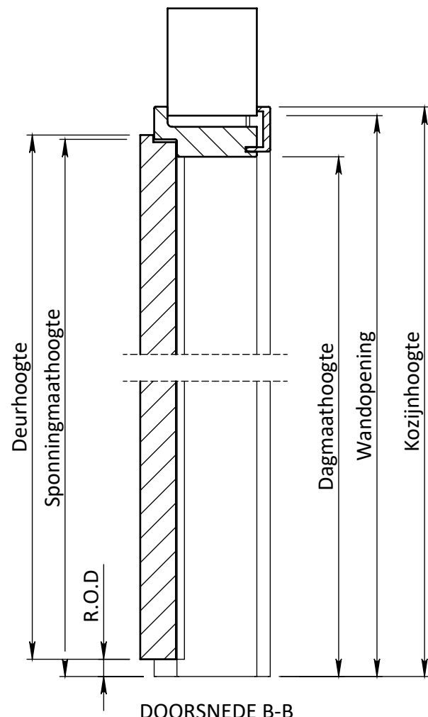
DOORSNEDE B-B
