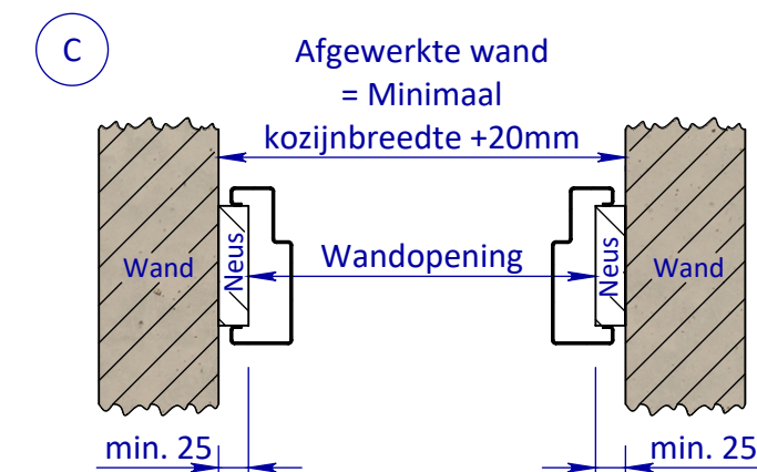
Kozijn tweezijdig niet wandomvattend
