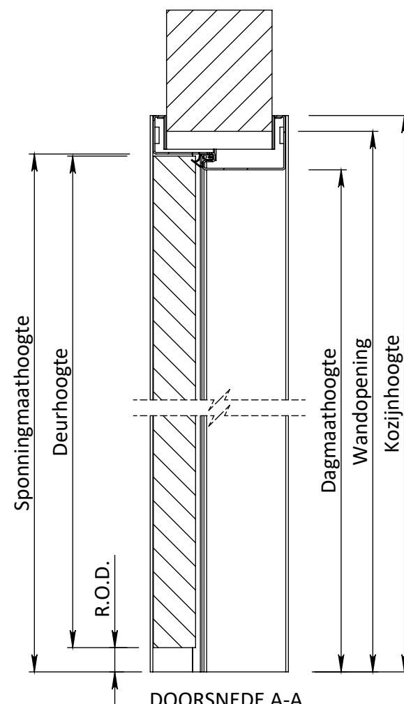
DOORSNEDE A-A
