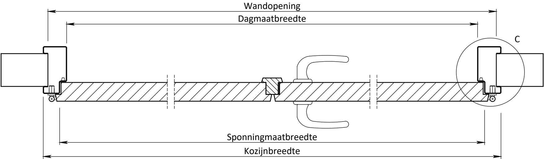
DOORSNEDE A-A
