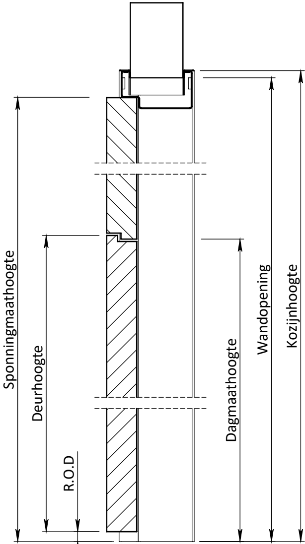
DOORSNEDE B-B
