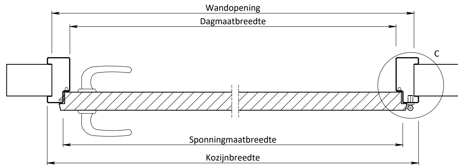
DOORSNEDE A-A
