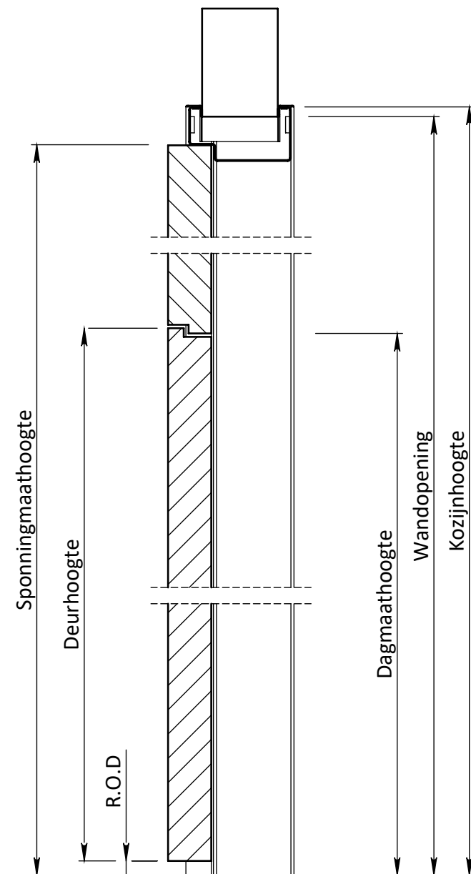
DOORSNEDE B-B
