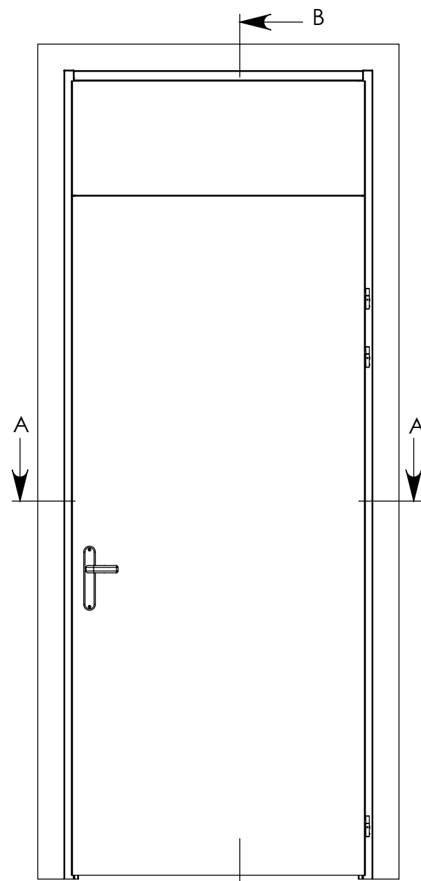
VOORAANZICHT
